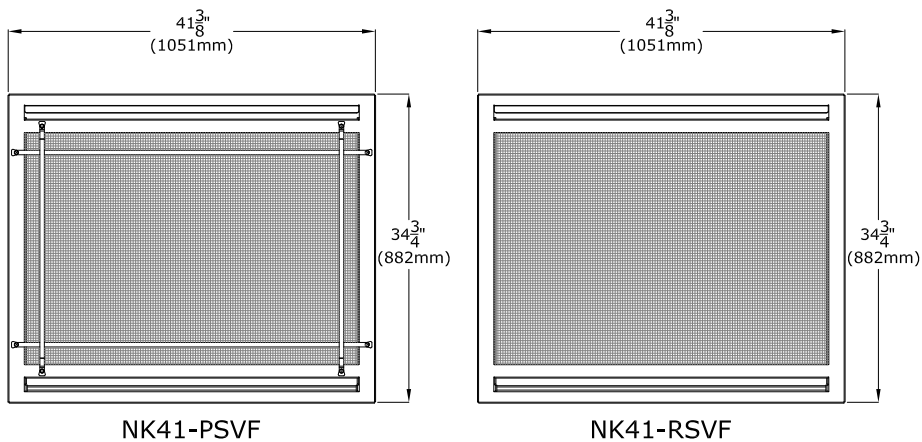
Figure 2.2 - Écrans pare-étincelles (Groupe 1)
