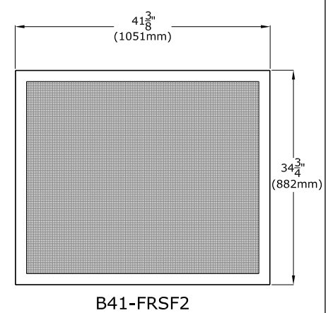
Figure 2.3 - Écrans pare-étincelles (Groupe 2)
