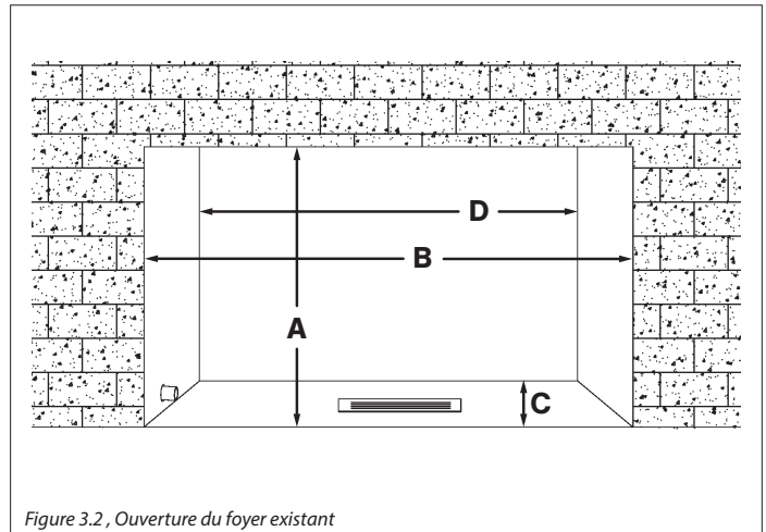
Figure 3.2, Ouverture du foyer existant
