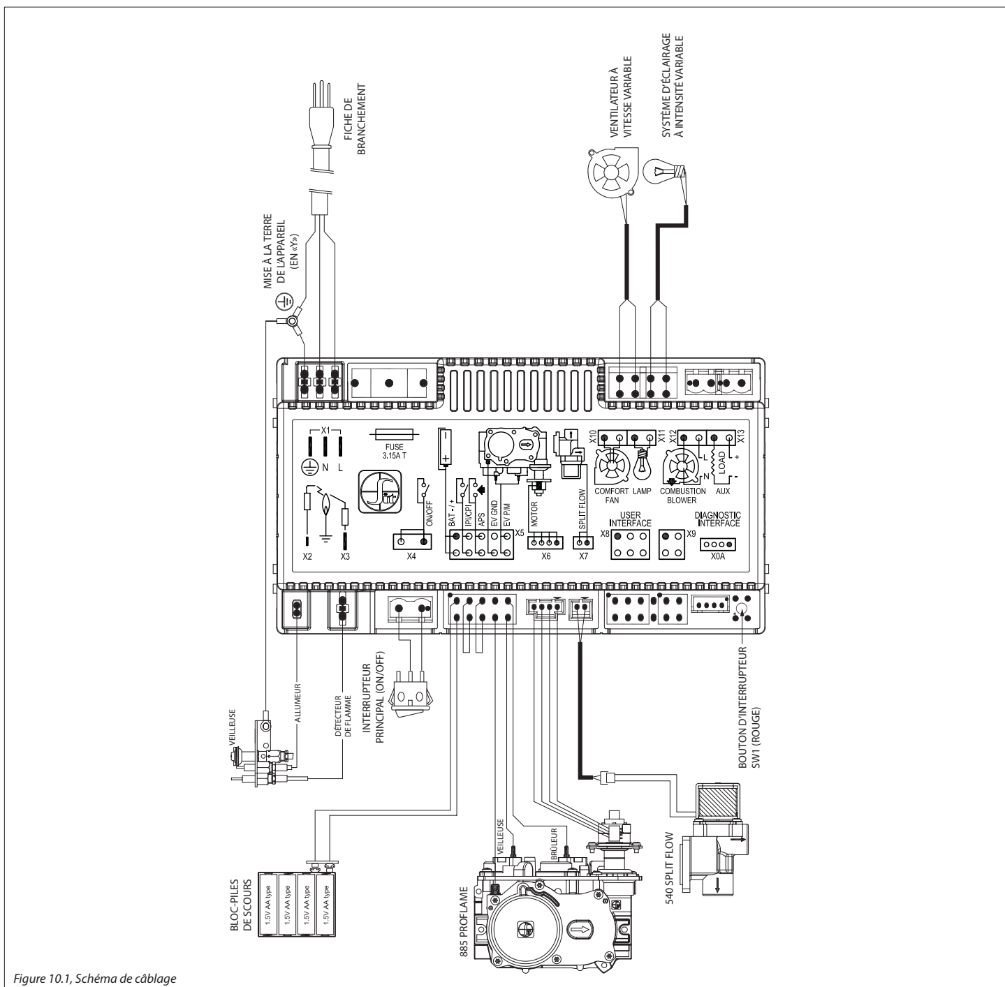
Figure 10.1, Schéma de câblage
