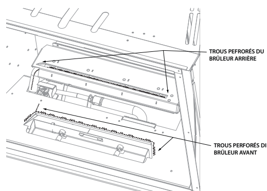
Figure 14.1, Système de brûleur et veilleuse
