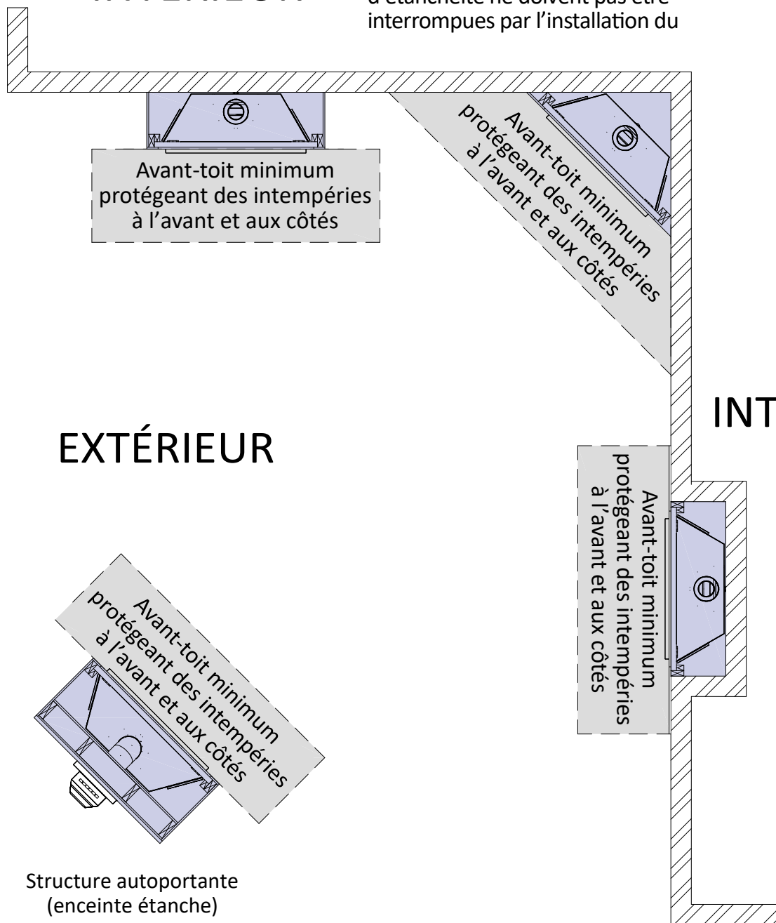
Figure 3.7 - Installation du foyer extérieur couvert
