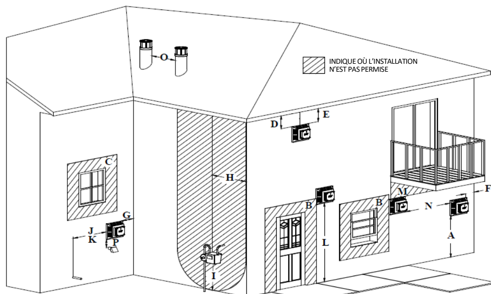
Figure 6.3 - Dégagements des terminaisons d'évacuation
