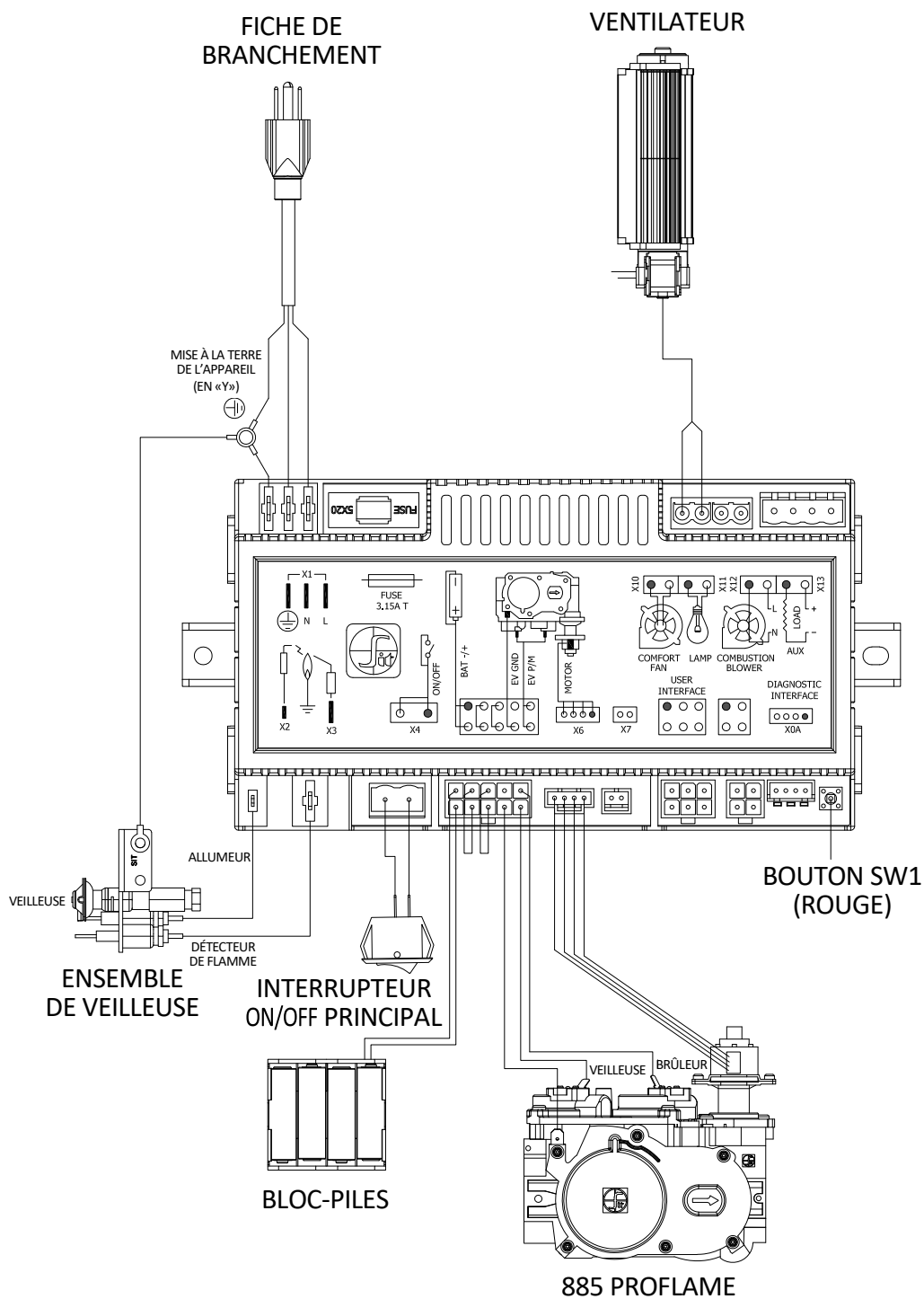
Figure 9.1 - Schéma électrique du SP-41-L
