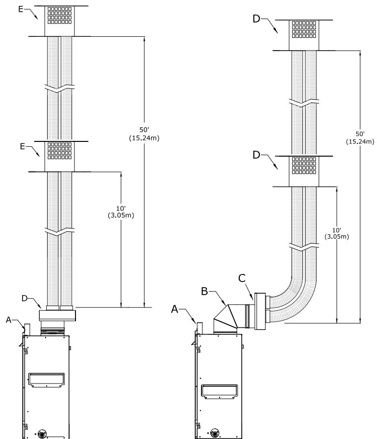
Figure 7.7 - Conduits de cheminée coaxiaux à colinéaires
