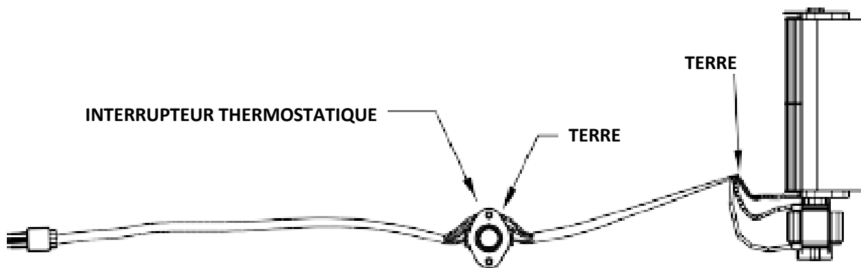
Figure 8.8 - Interrupteur thermostatique
