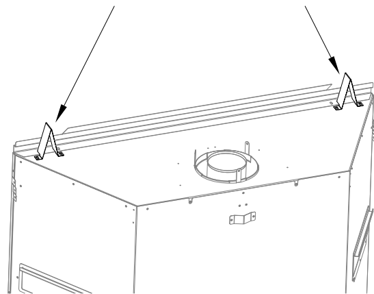
Figure 3.1 - Installation des étriers de dégagement
