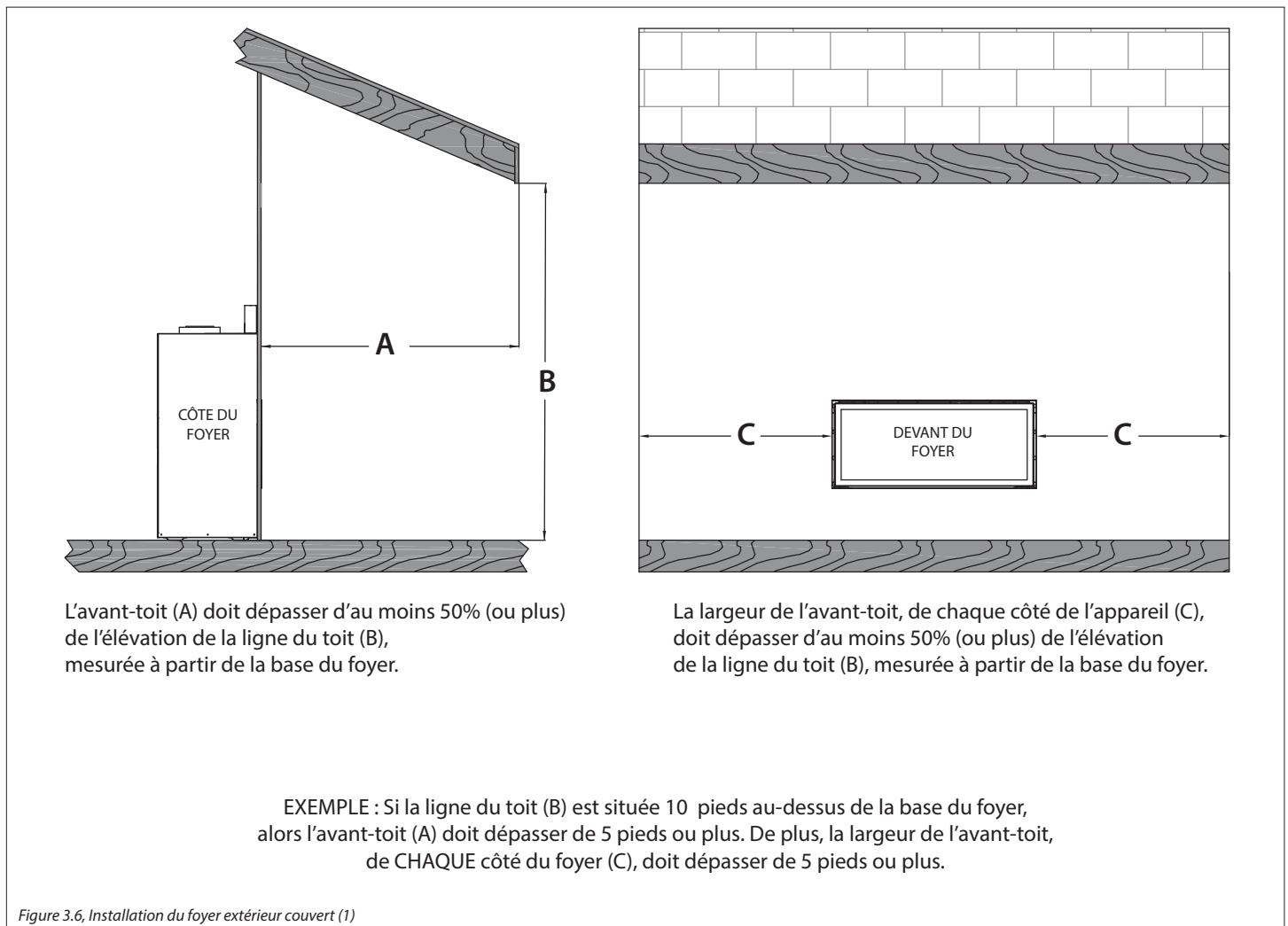
Figure 3.6, Installation du foyer extérieur couvert (1)
