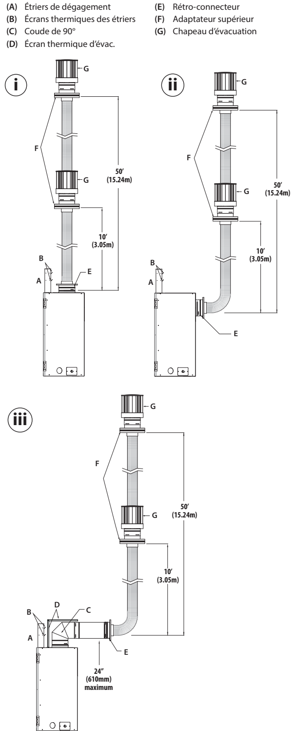
SCHÉMA 6 CONVERSION DE CHEMINÉE AVEC CONDUIT FLEXIBLE 4 PO
