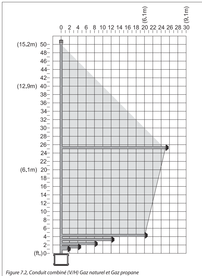
Figure 7.2, Conduit combiné (V/H) Gaz naturel et Gaz propane
