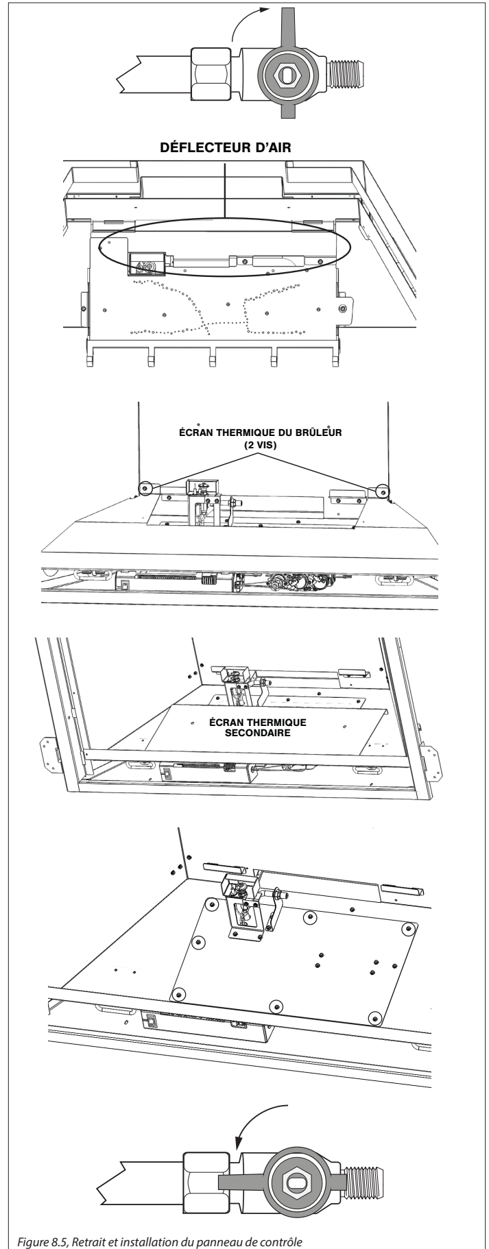
Figure 8.5, Retrait et installation du panneau de contrôle
