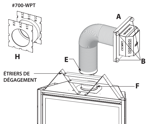
Figure 7.5, Assemblage et installation du kit de terminaison (Série n° 700-2)
