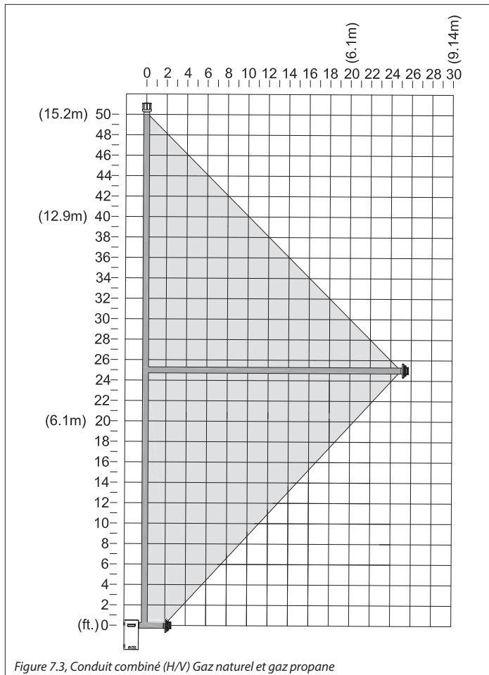
Figure 7.3, Conduit combiné (H/V) Gaz naturel et gaz propane
