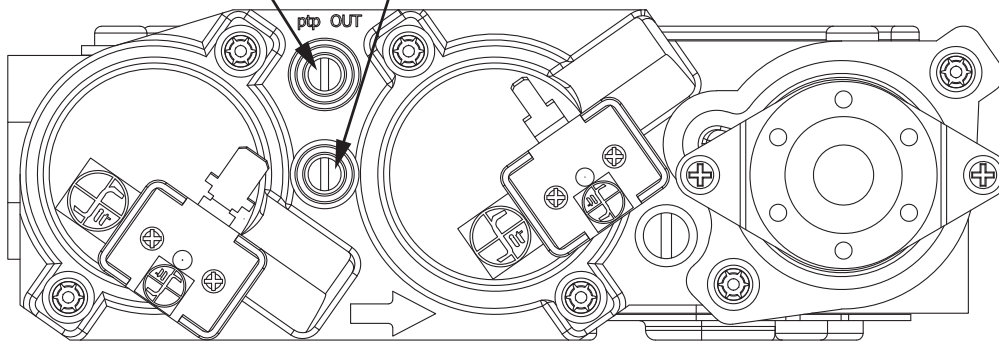
Figure 11.1, Raccords de test pression de valve de contrôle de gaz
