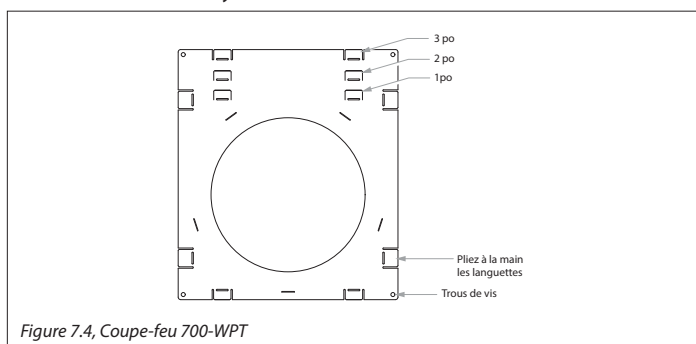
Figure 7.4, Coupe-feu 700-WPT
