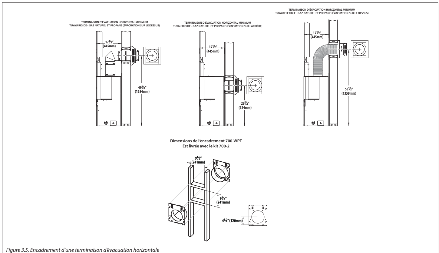
Figure 3.5, Encadrement d'une terminaison d'évacuation horizontale
