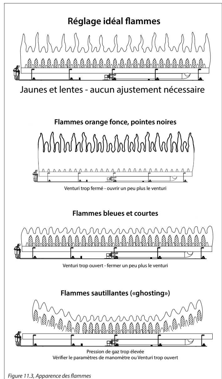
Figure 11.3, Apparence des flammes
