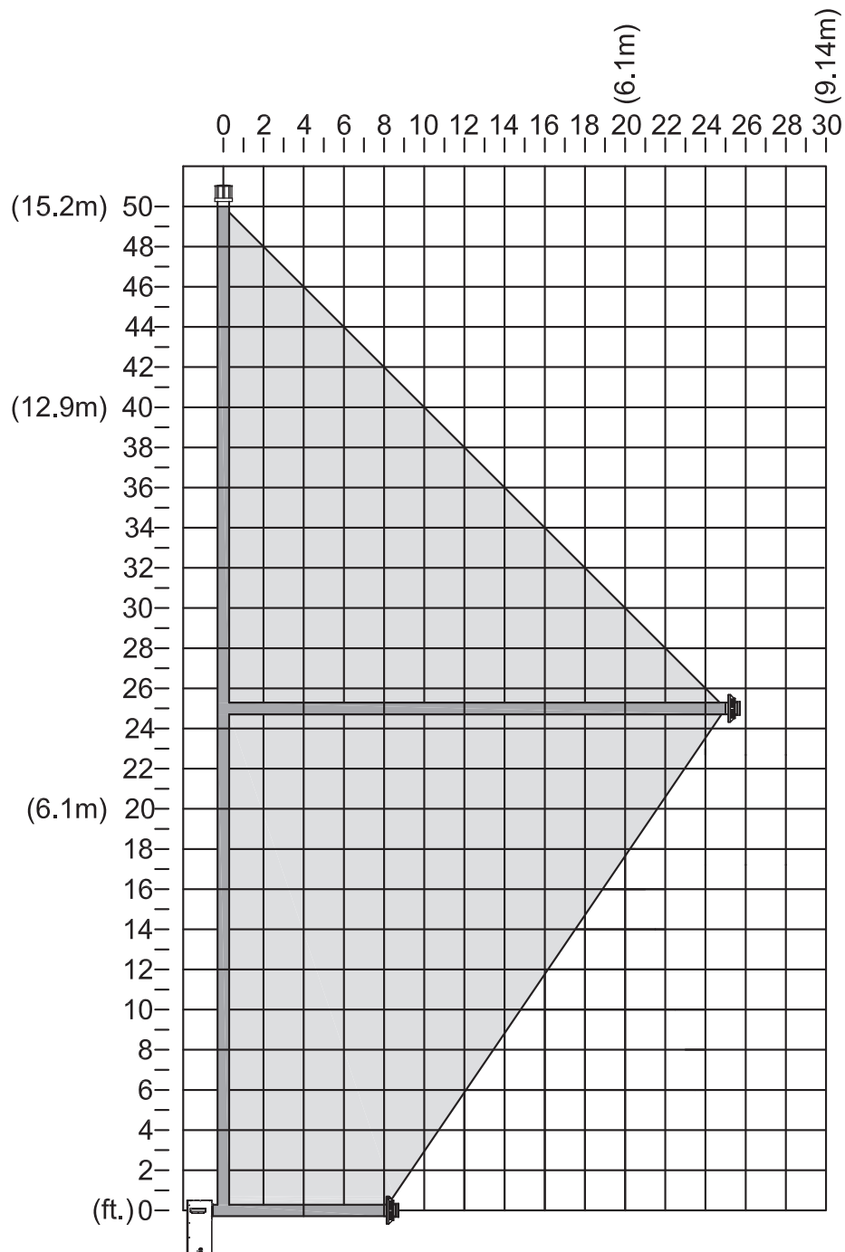
Figure 7.6, Conduit combiné (H/V) Gaz naturel SUELEMENT
